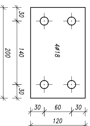
Poz.384, 136x, S355J2 Plate 12x120x200
